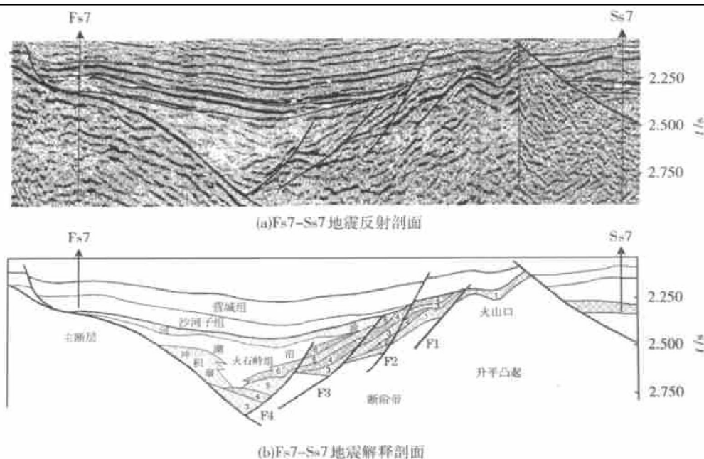
图2 构造断阶带与火山岩体及地层结构
